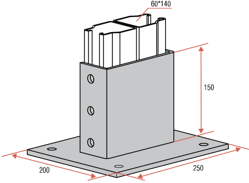
PLGBB.86140
