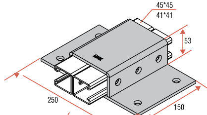
PLGBB.8633 PLGBB.6633
