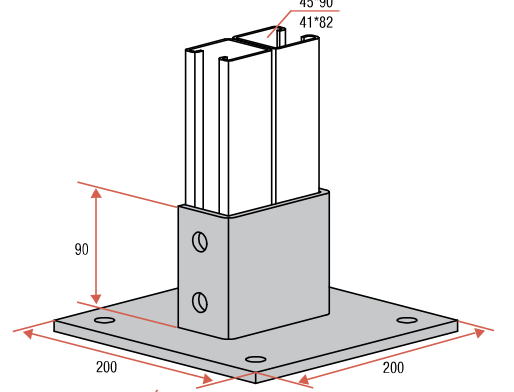
PLGBB.8690 PLGBB.6690
