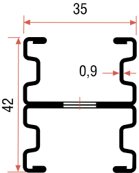
PLC 35 x 42 x 0,9
