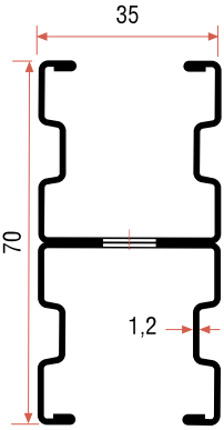
PLC 35 x 70 x 1,2
