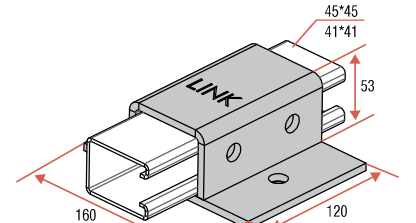
PLGBB.8631 PLGBB.6631
