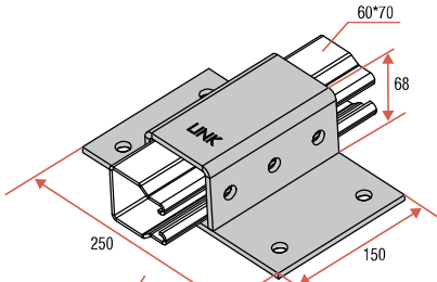
PLGBB.8632 PLGBB.6632
