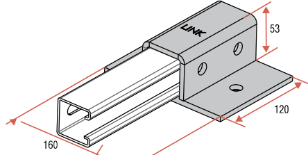
PLGBB.8630 PLGBB.6630
