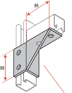
PLGYBF.8546 PLGYBF.6546
