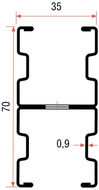
PLC 35 x 70 x 0,9
