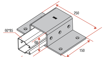
PLGBB.8634
