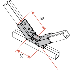
PLGYBF.8562 PLGYBF.6546
