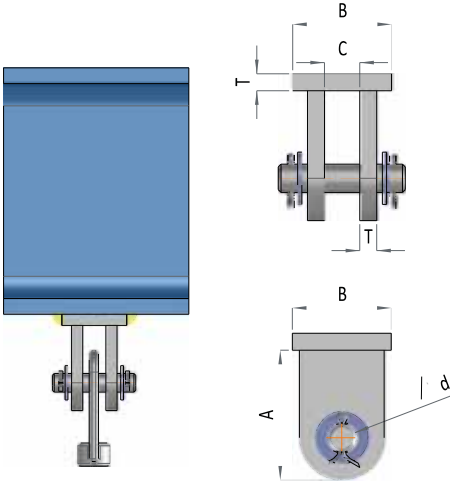
KAYNAKLI MAŞA / WELD ON CLEVIS
