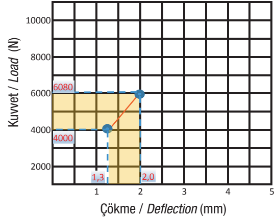
Kuvvet-Çökme Grafiği / Load - Deflection Table
